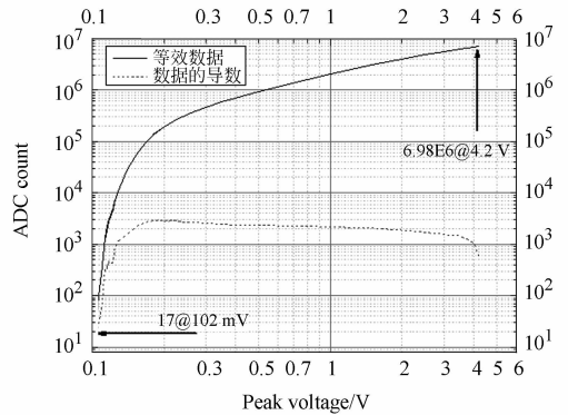
(b) 等效数据输出
