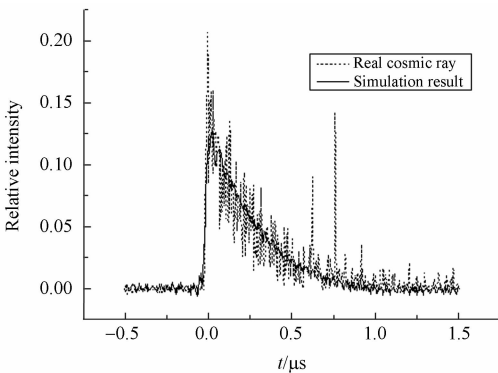
图 7 波形匹配度对比 Fig. 7 Waveform matching
