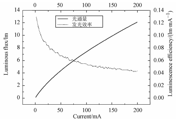
图 3 选用 LED 的电流/光通量曲线
