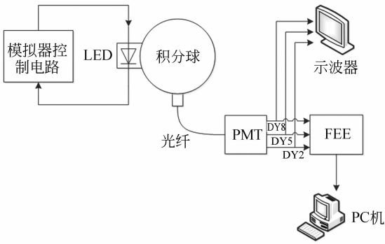
图 6 测试装置示意图 Fig. 6 Scheme of test system
