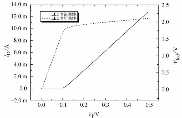
图5 分流电路伏安曲线示意图
